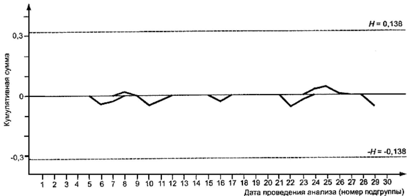
Рисунок 10 - Контрольная карта кумулятивных сумм для оценки \hat{\delta} - систематической погрешности определения зольности, % (по массе) собственного стандартного образца
