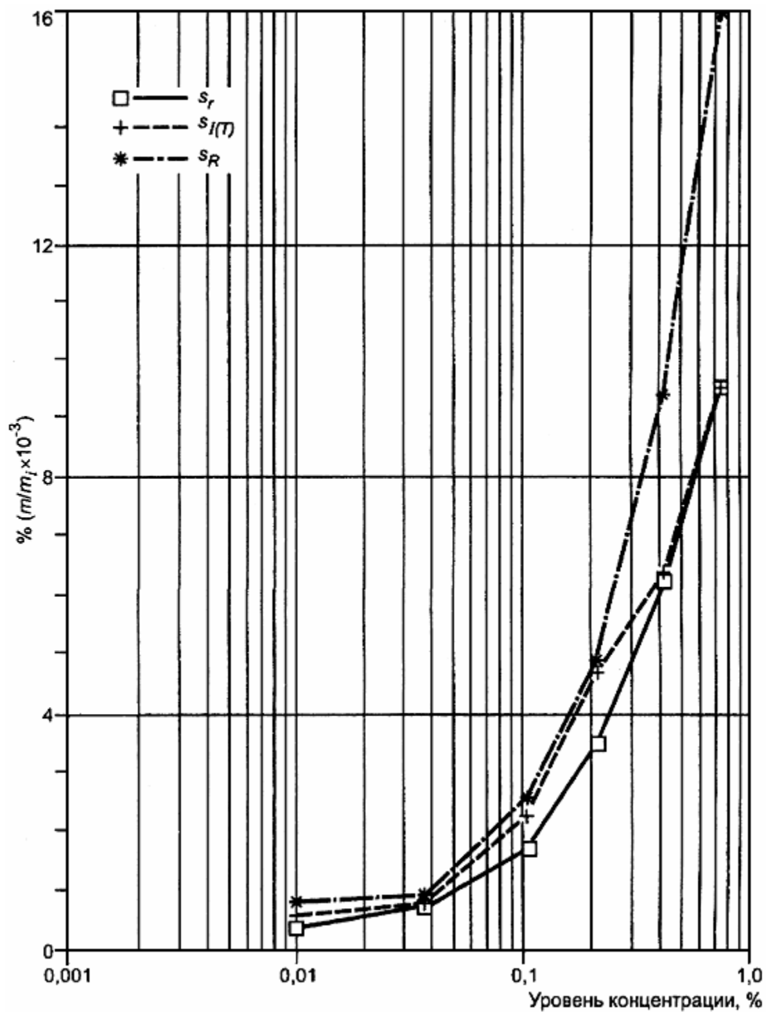
Рисунок D.3 - Содержание ванадия в стали. Стандартные отклонения повторяемости s_r , промежуточной
