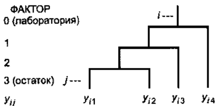
Рисунок 2 - Схема четырехфакторного ступенчато вложенного эксперимента
