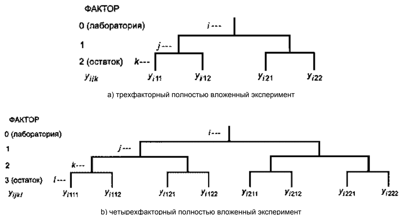
Рисунок 1 - Схемы трех- и четырехфакторных полностью вложенных экспериментов
