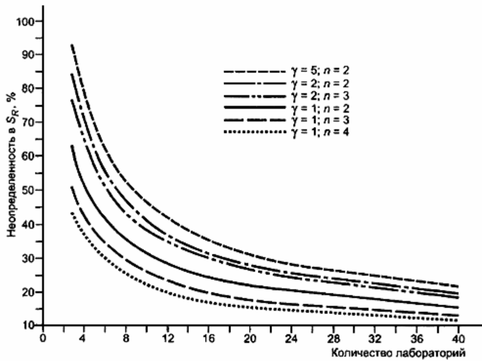
Рисунок В.2 - Ожидаемая величина, на которую \hat{S}_R может отличаться от истинного значения на уровне
