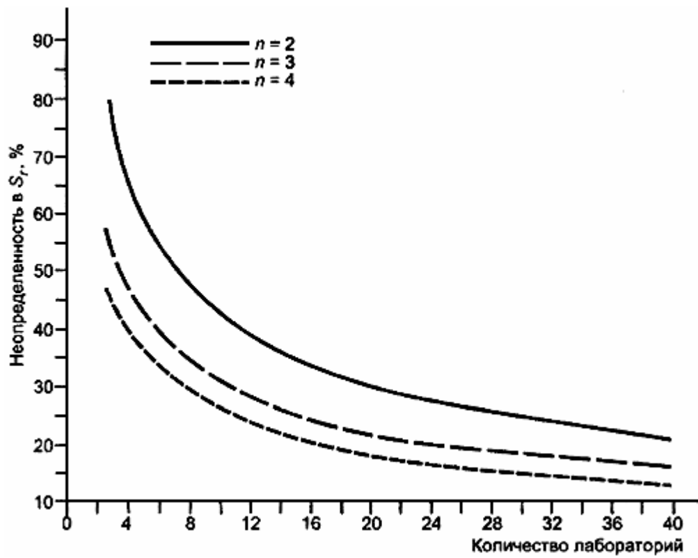
Рисунок В.1 - Ожидаемая величина, на которую \hat{S}_r может отличаться от истинного значения на уровне вероятности 95%
